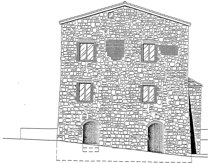
PROSPETTO SUD
