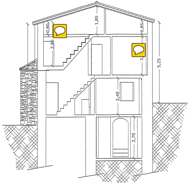
SEZIONE
