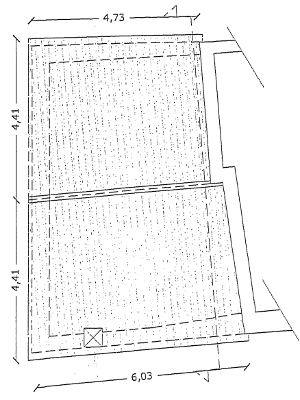
PIANTA COPERTURA
