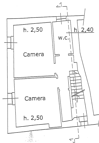
PIANO PRIMO
